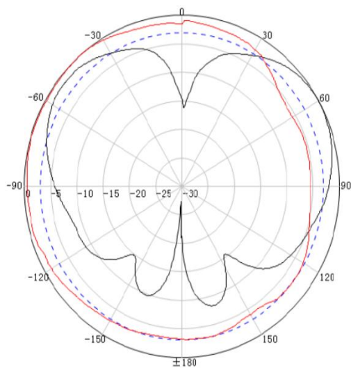
1710MHz
