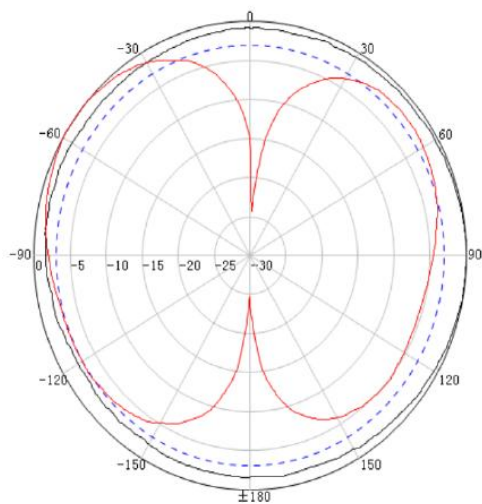
698MHz
