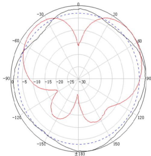
960MHz
