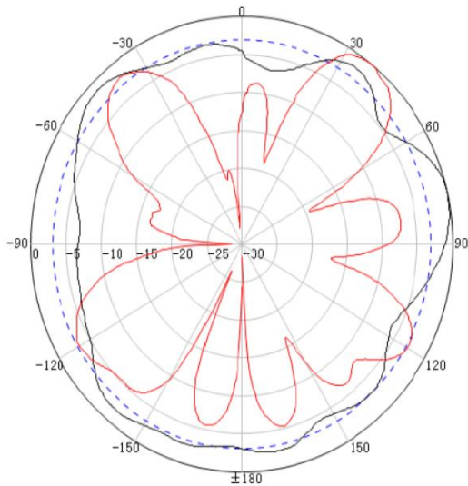
2700MHz
